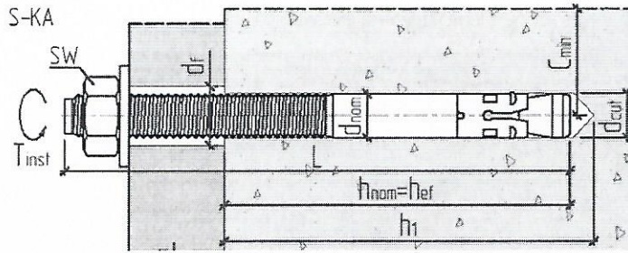
Рис. 2. Установочные параметры анкеров S-KA
