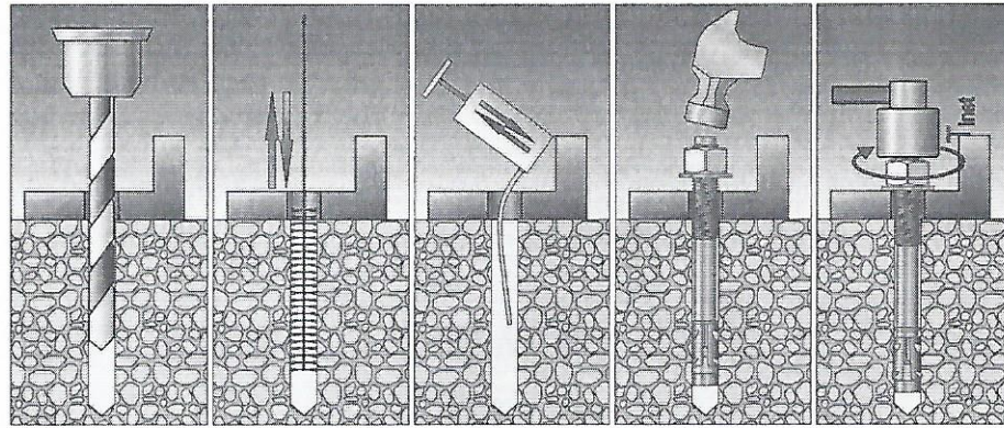
Рис. 3. Установка анкеров S-KA
